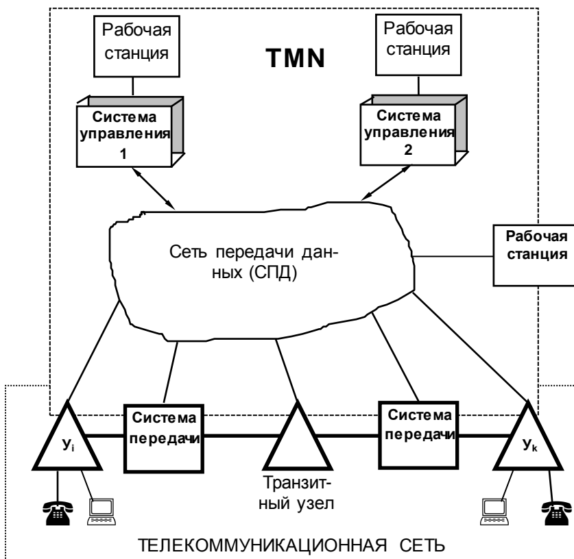
Рисунок 9.2. Взаимодействие СУ с телекоммуникационной сетью
