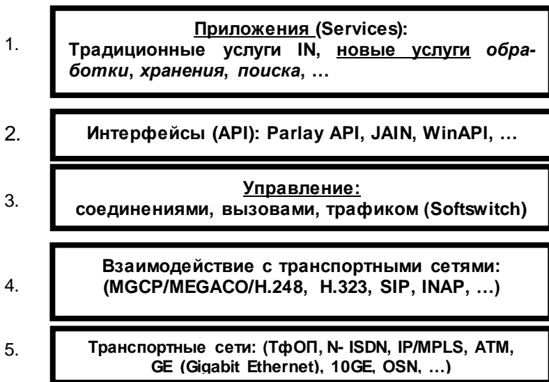
Рисунок 4.5. Функции уровней и протоколы NGN
