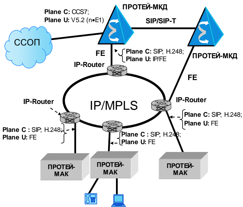
Рисунок 10.14. Схема мультисервисной сети, построенной с помощью оборудования НТЦ ПРОТЕЙ
