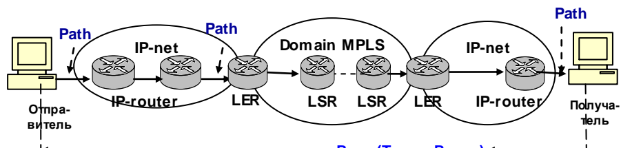
Рисунок 5.3 – Запрос характеристик качества доставки данных
