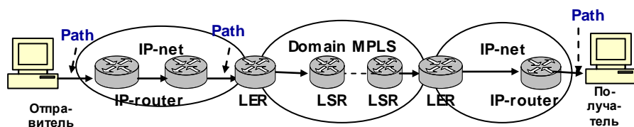
Рисунок 5.2 – Запрос характеристик качества доставки данных
