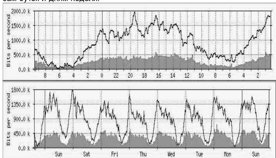
Рисунок 10.1. Графики загрузки интерфейса E1 потоками пакетов с компрессированной речевой информацией по часам суток и дням недели. Из графиков на рисунке 10.1 видно, что соотношение между пиковыми объемами передаваемой информации и средним объемом передаваемой информации является величиной достаточно стабильной, лежащей в диапазоне 2-3. В расчетах можно принять это соотношение равным 2,5.
