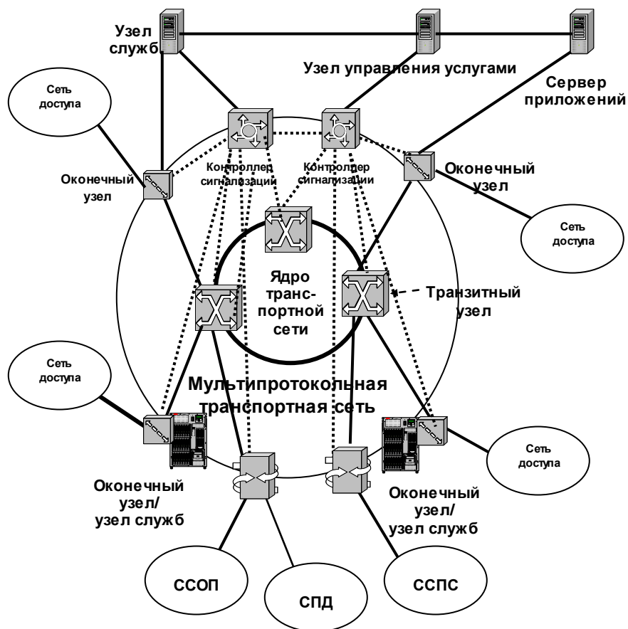
Рисунок 5.5. Архитектура NGN
