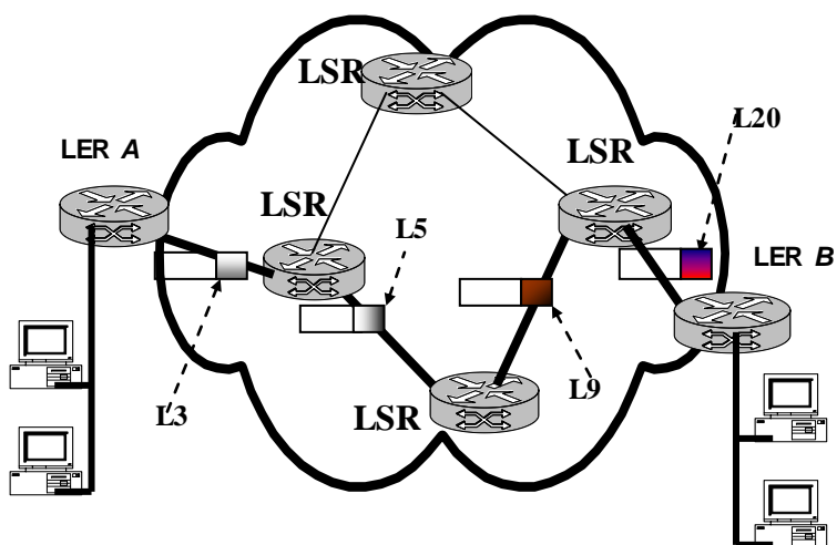
Рисунок 7.9 – Метки, уникальные в каждом звене, используются для коммутации пакетов в домене MPLS
